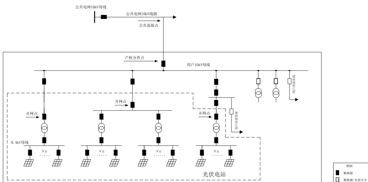
图 19-4 XGF10-Z-Z1 方案原则电气主接线图（方案二）
