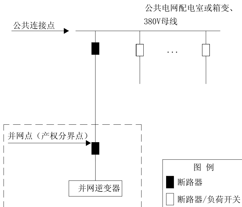
图 5-6 XGF380-T-2 方案一次系统接线示意图
