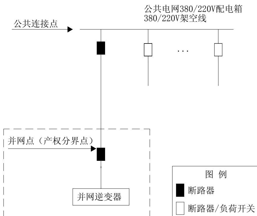
图 5-5 XGF380-T-1 方案一次系统接线示意图
