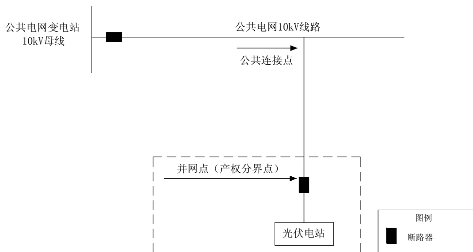
图 5-3 XGF10-T-3 方案一次系统接线示意图
