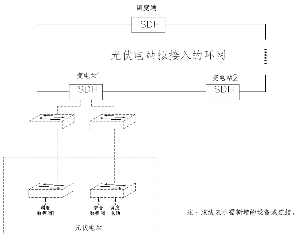
图 19-12 光伏电站接入系统方案图 2（工业以太网）
