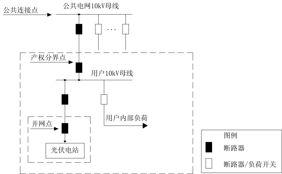
图 5-4-1 XGF10-Z-1 方案一次系统接线示意图（方案一）
