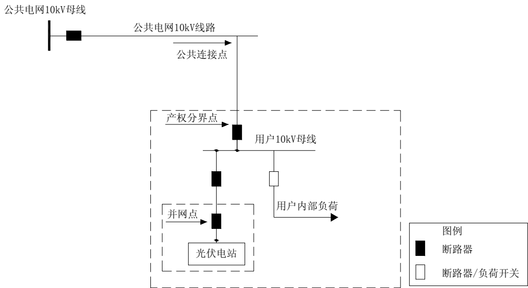
图 5-4-2 XGF10-Z-1 方案一次系统接线示意图（方案二）
