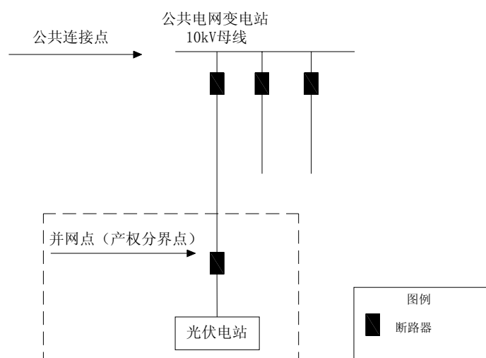
图 5-1 XGF10-T-1 方案一次系统接线示意图
