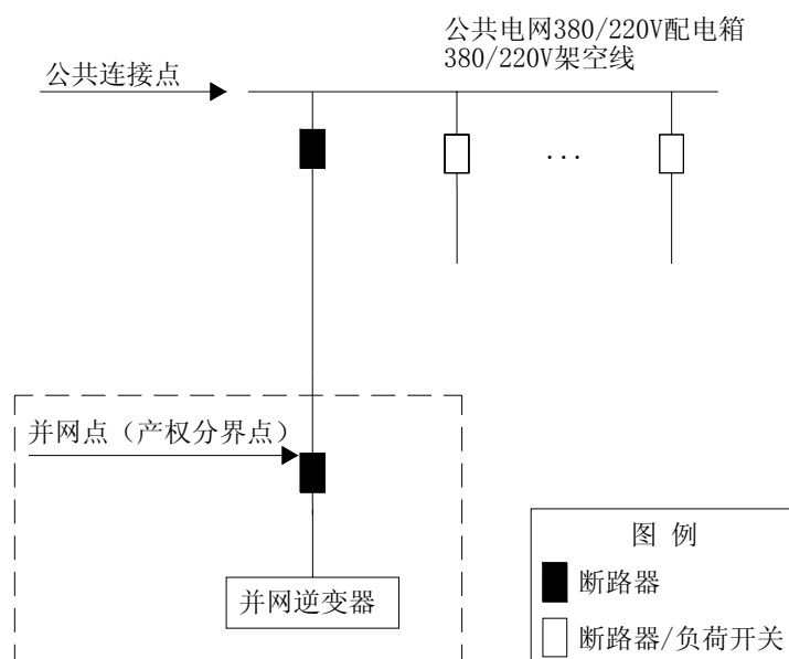
图 14-1 XGF380-T-1 方案一次系统接线示意图
