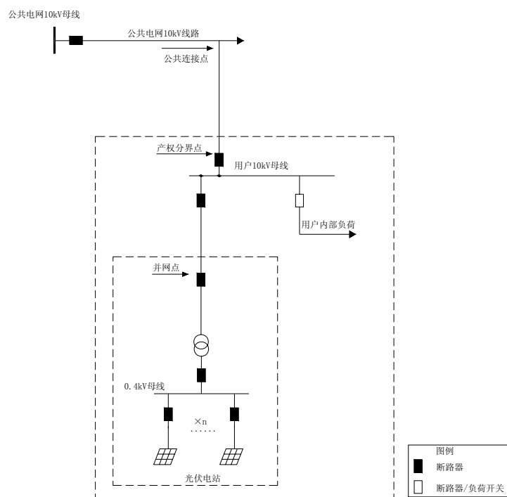
图 13-4 XGF10-Z-1 方案原则电气主接线图（方案二）
