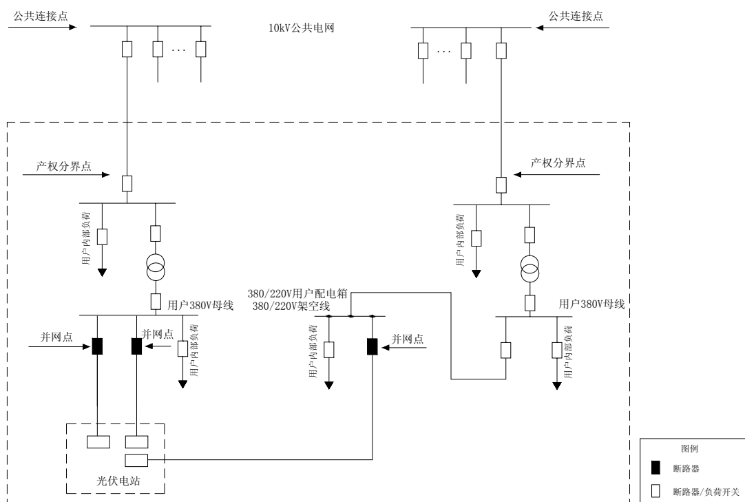
图 18-1 XGF380-Z-Z1 方案一次系统接线示意图（方案一）
