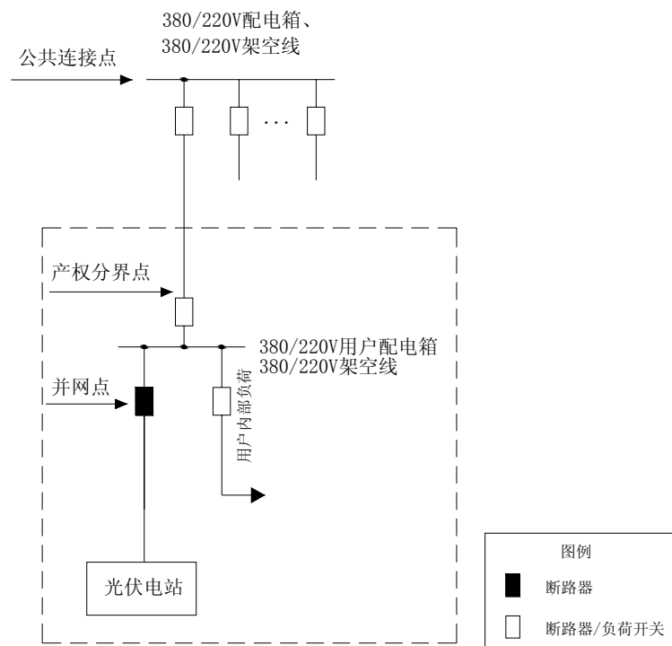
图 5-7-1 XGF380-Z-1 方案一次系统接线示意图（方案一）
