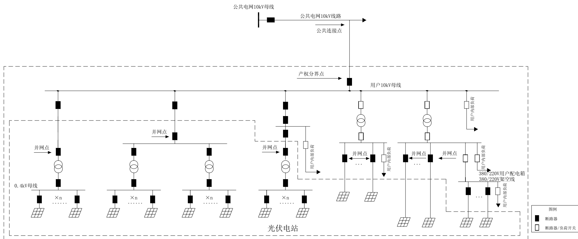
图 20-4 XGF380/10-Z-Z1 方案原则电气主接线图（方案二）
