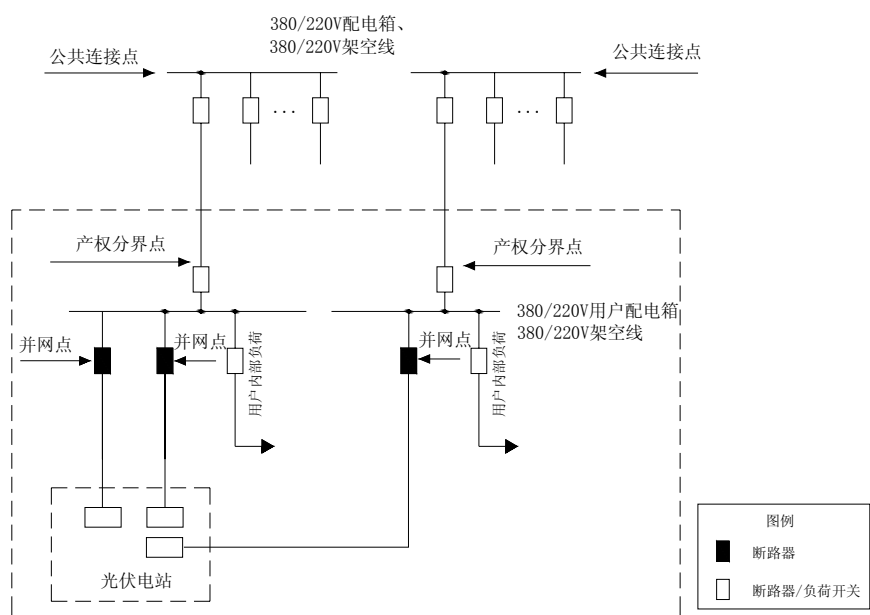
图 5-9-1 XGF380-Z-Z1 方案一次系统接线示意图（方案一）
