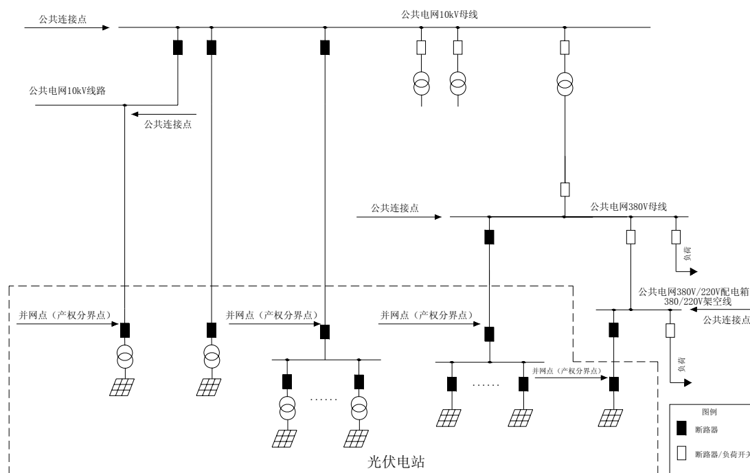
图 22-2 XGF380/10-T-Z1 方案原则电气主接线图
