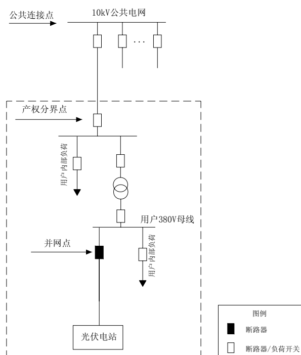
图 5-8 XGF380-Z-2 方案一次系统接线示意图
