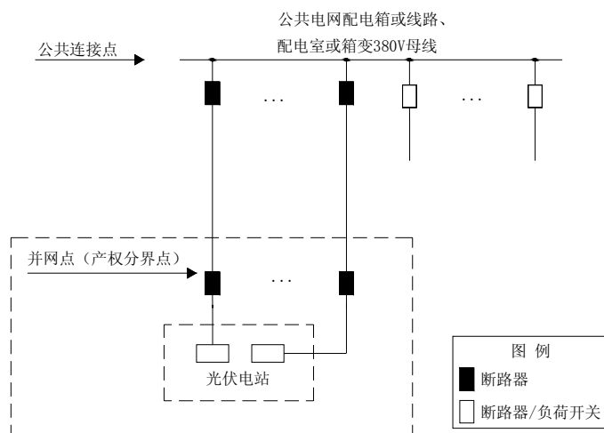
图 21-1 XGF380-T-Z1 方案一次系统接线示意图
