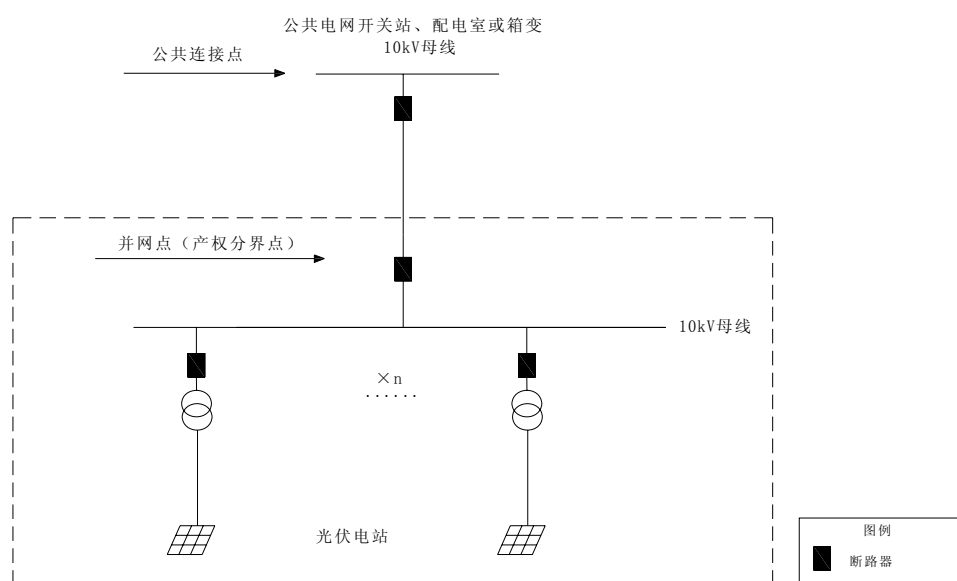
图 11-2 XGF10-T-2 方案原则电气主接线图（方案一）
