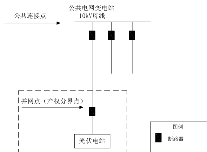
图 10-1 XGF10-T-1 方案一次系统接线示意图
