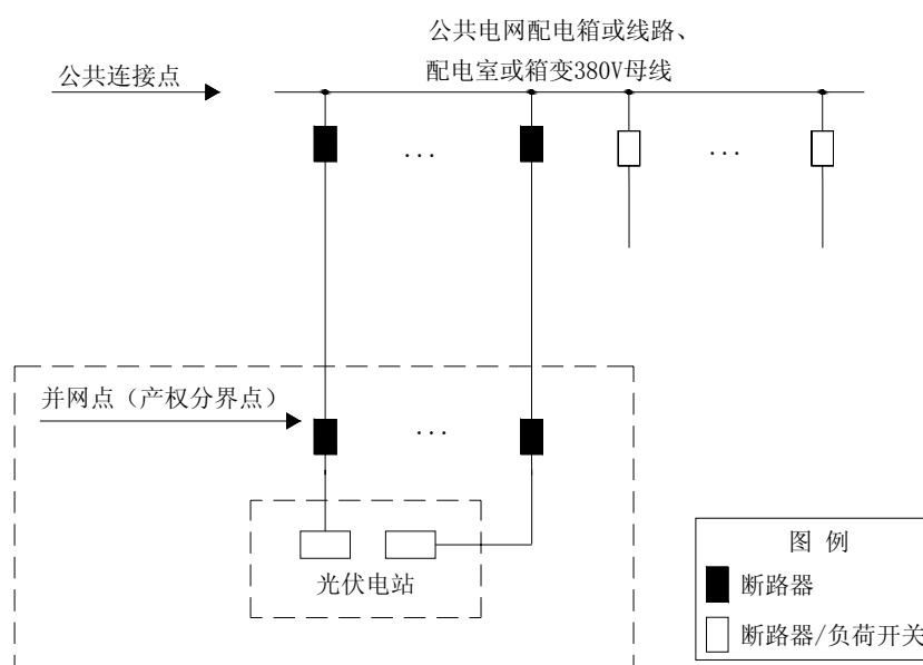
图 5-12 XGF380-T-Z1 方案一次系统接线示意图
