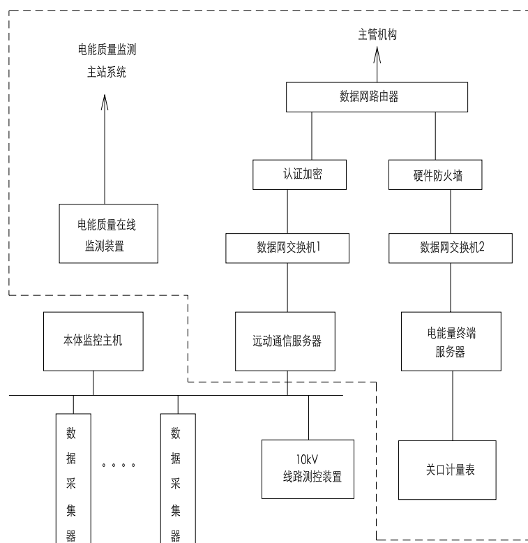
图 22-5 XGF380/10-T-Z1 光伏电站调度自动化系统图（方案一）
