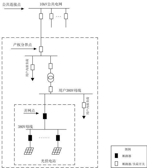
图 17-2 XGF380-Z-2 方案原则电气主接线图
