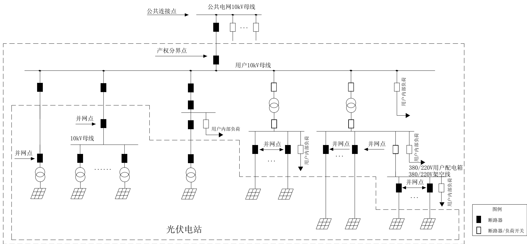
图 20-3 XGF380/10-Z-Z1 方案原则电气主接线图（方案一）
