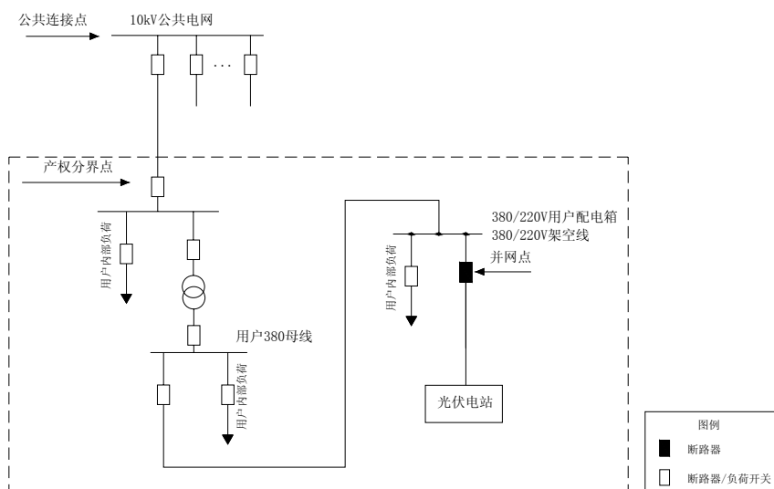
图 5-7-2 XGF380-Z-1 方案一次系统接线示意图（方案二）
