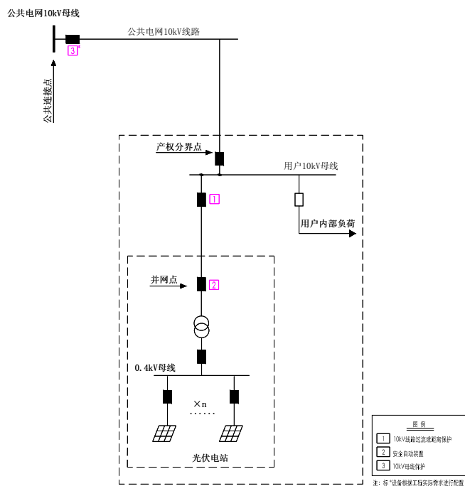
图 13-6 XGF10-Z-1 系统继电保护及安全自动装置配置(方案一/2 )
