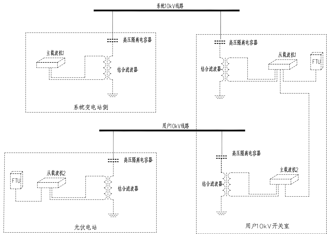
图 19-14 光伏电站接入系统方案图（中压电力线载波）
