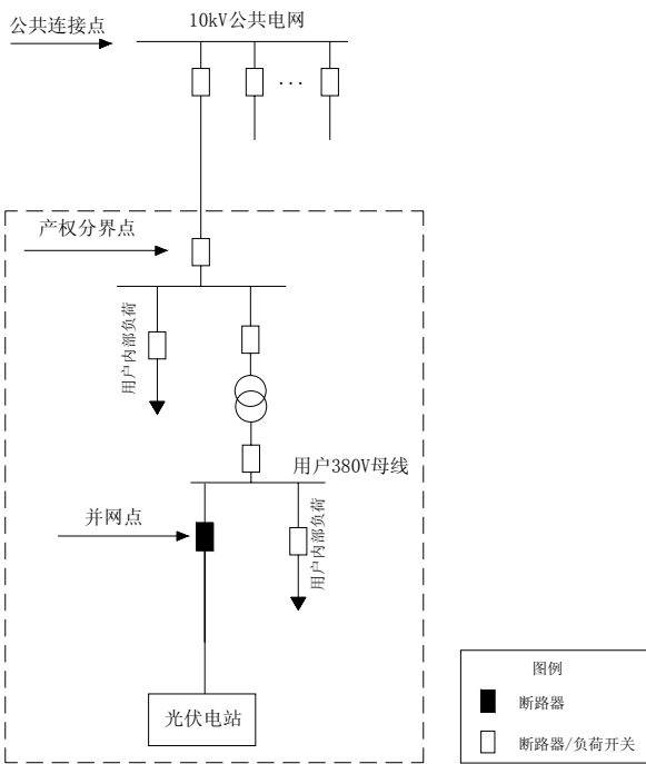
图 17-1 XGF380-Z-2 方案一次系统接线示意图
