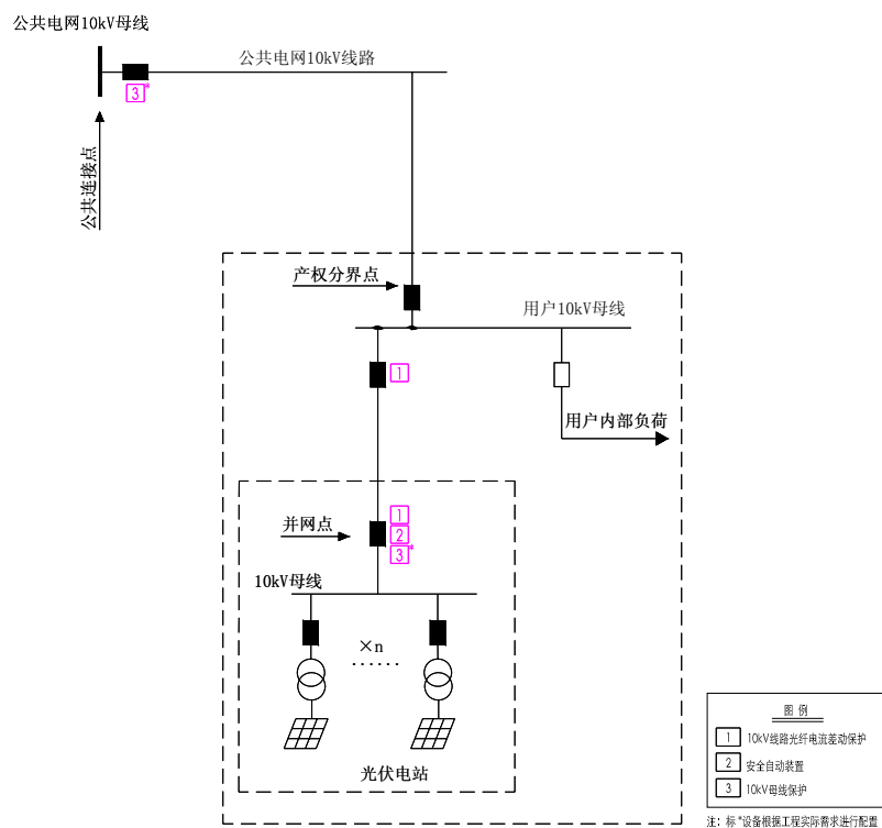
图 13-8 XGF10-Z-1 系统继电保护及安全自动装置配置(方案二/2 )
