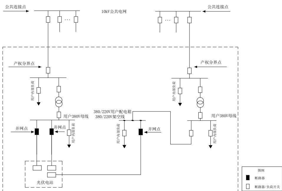
图 5-9-2 XGF380-Z-Z1 方案一次系统接线示意图（方案二）
