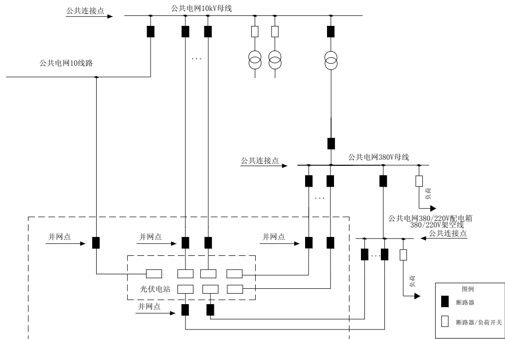
图 5-13 XGF380/10-T-Z1 方案一次系统接线示意图
