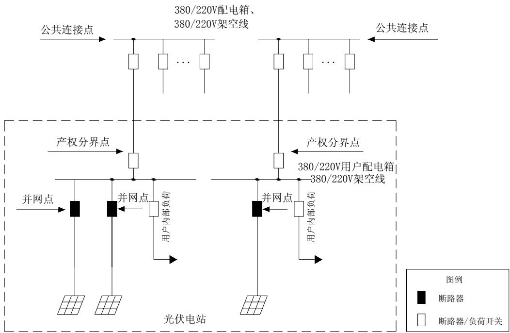
图 18-3 XGF380-Z-Z1 方案原则电气主接线图（方案一）
