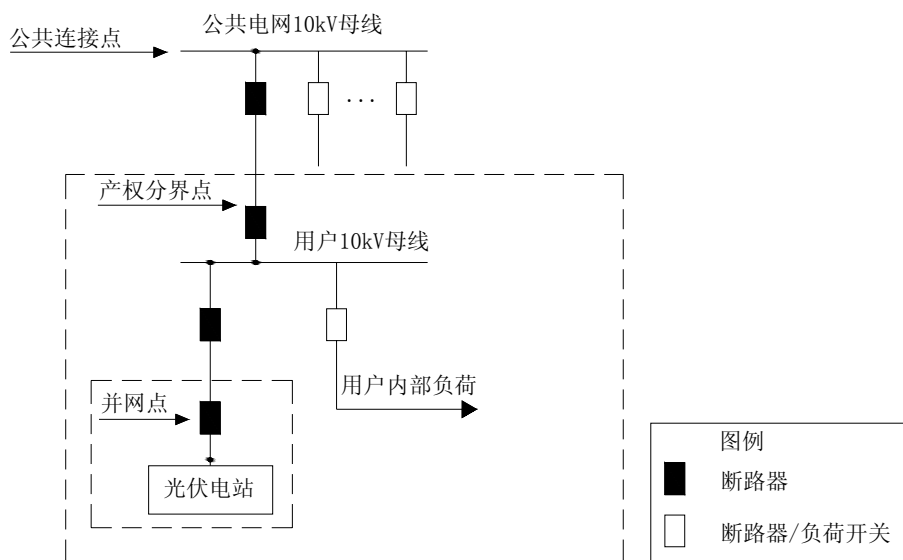
图 13-1 XGF10-Z-1 方案一次系统接线示意图（方案一）
