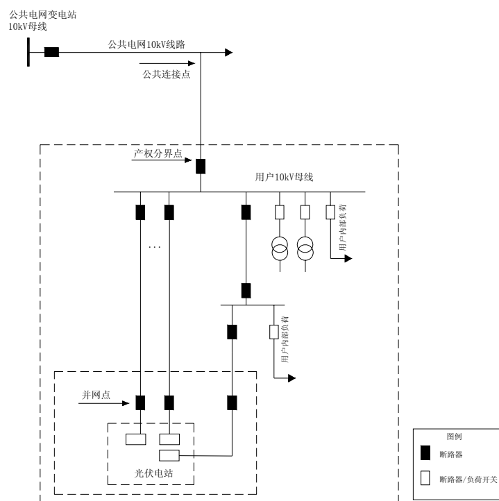
图 5-10-2 XGF10-Z-Z1 方案一次系统接线示意图（方案二）
