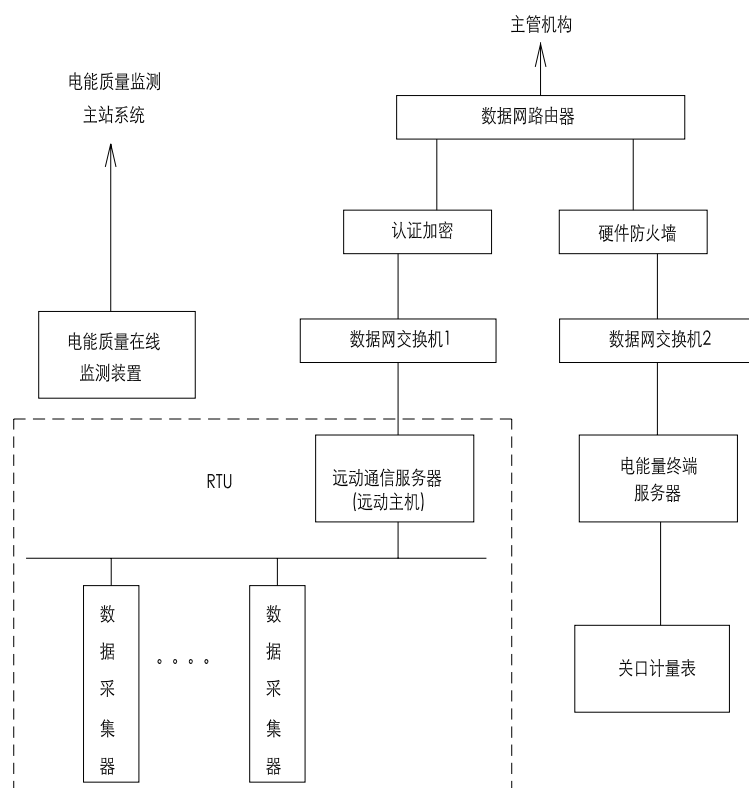
图 19-9 XGF10-Z-Z1 光伏电站调度自动化系统配置（方案一）
