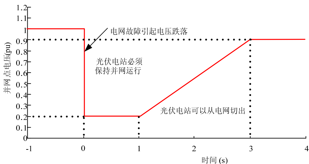
图 4-1 大中型光伏电站的低电压穿越能力要求
