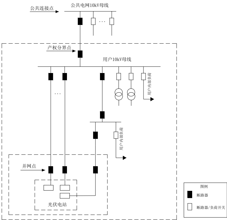
图 5-10-1 XGF10-Z-Z1 方案一次系统接线示意图（方案一）
