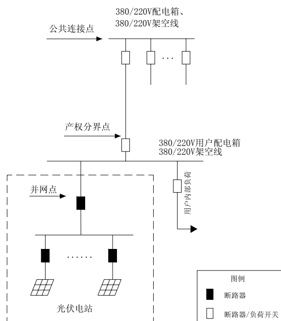
图 16-3 XGF380-Z-1 方案原则电气主接线图（方案一）
