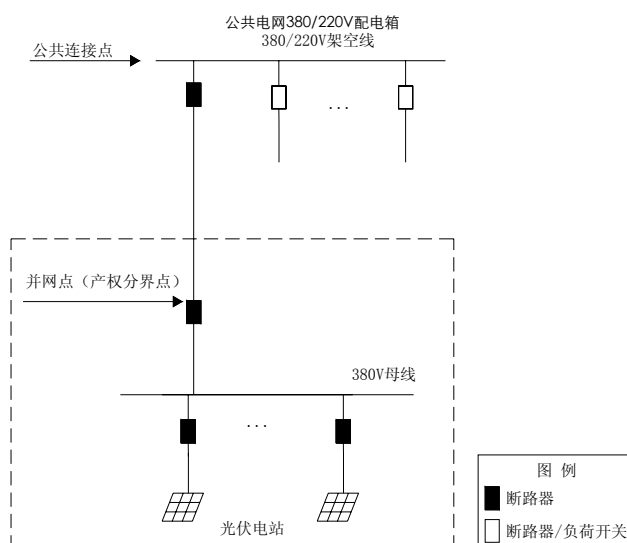
图 14-2 XGF380-T-1 方案原则电气主接线图
