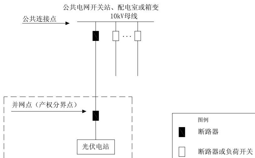
图 5-2 XGF10-T-2 方案一次系统接线示意图
