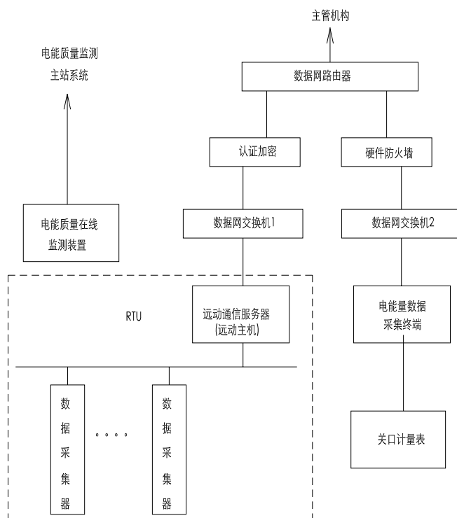
图 20-10 XGF380/10-Z-Z1 光伏电站调度自动化系统图（方案二）
