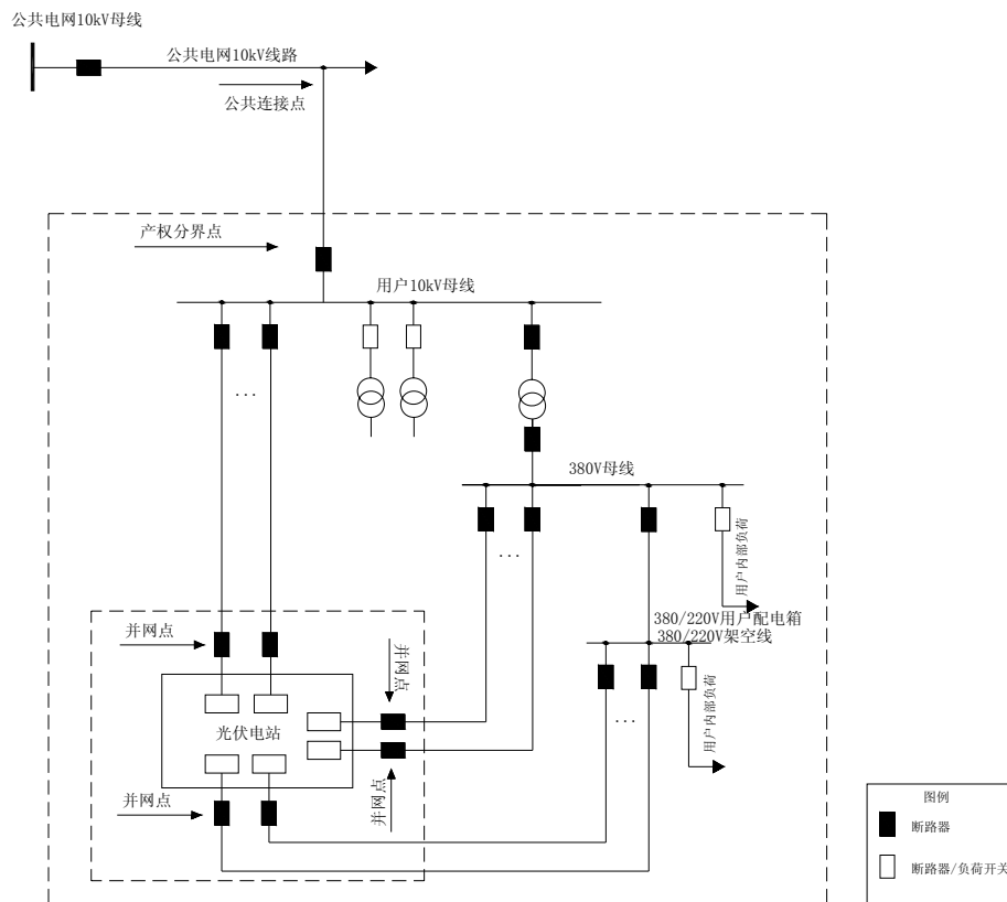
图 5-11-2 XGF380/10-Z-Z1 方案一次系统接线示意图（方案二）
