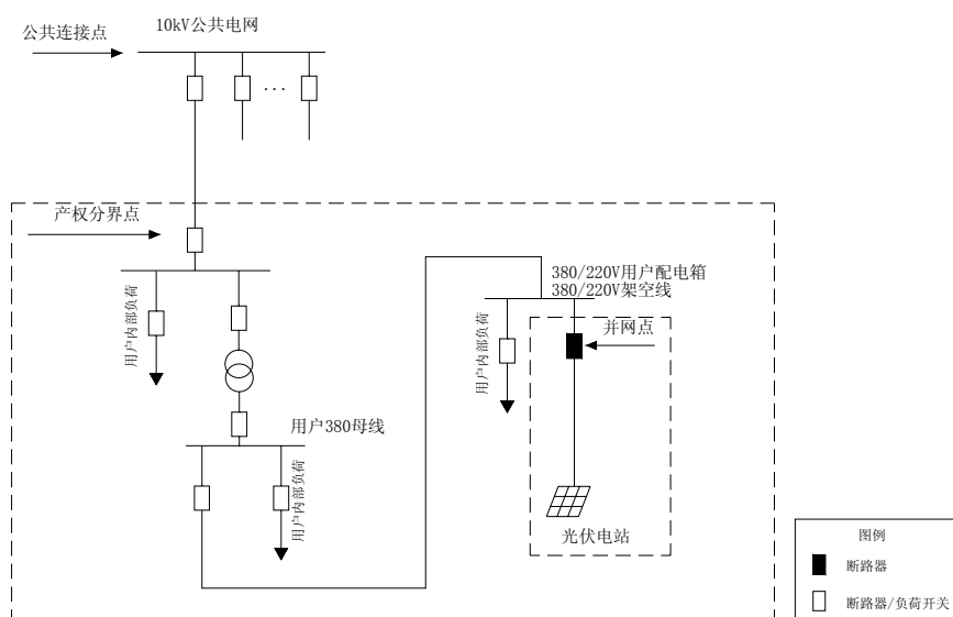
图 16-4 XGF380-Z-1 方案原则电气主接线图（方案二）
