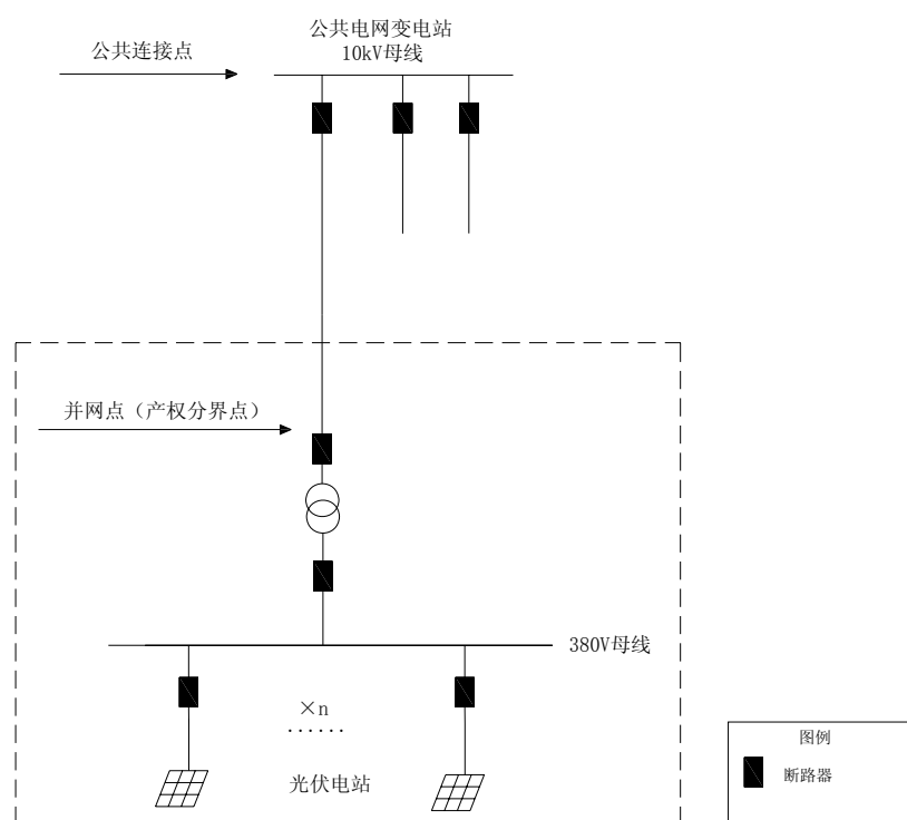
图 10-3 XGF10-T-1 方案原则电气主接线图（方案二）
