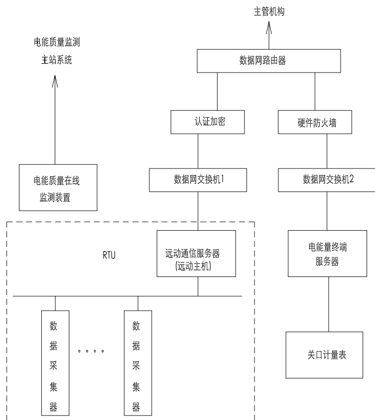
图 12-7 XGF10-T-3 光伏电站调度自动化系统配置（方案二）
