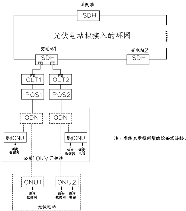
图 22-7 光伏电站接入系统方案图（EPON 公用 10kV 开关站（配电室）已实现配电自动化）
