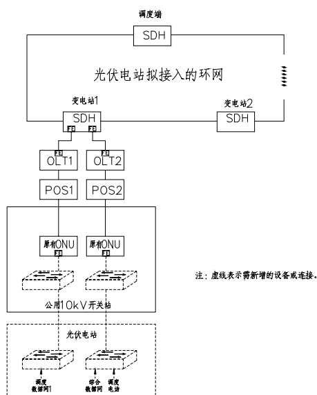
图 22-9 光伏电站接入系统方案图（工业以太网 10kV 开关站已实现配电自动化）
