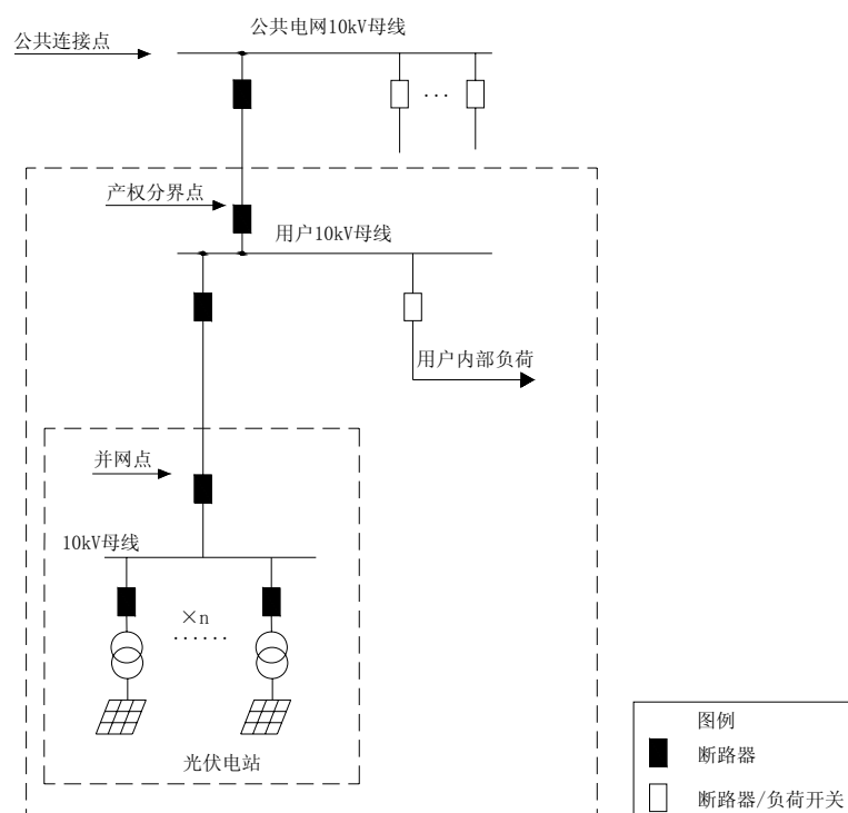
图 13-3 XGF10-Z-1 方案原则电气主接线图（方案一）
